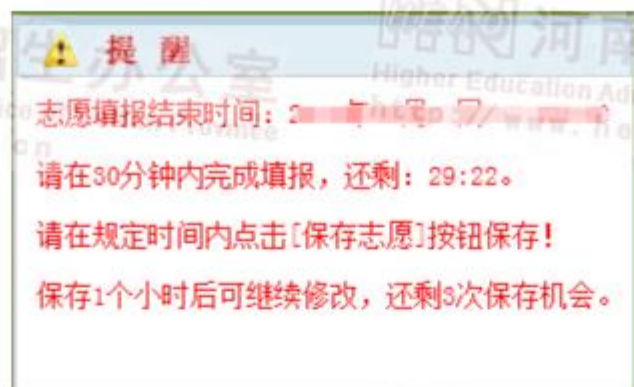
图 5 倒计时提醒
